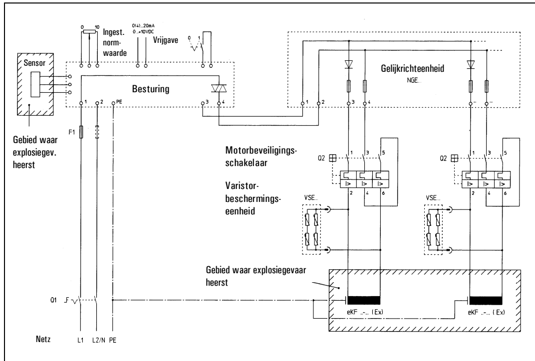
Afb. 4-5 Elektrisch schema, meervoudige aandrijving
